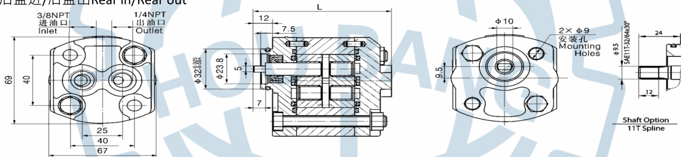
后盖进/前盖出 Rear in/front out
