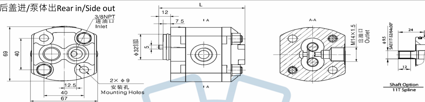
泵体进/泵体出 Side in/Side out
