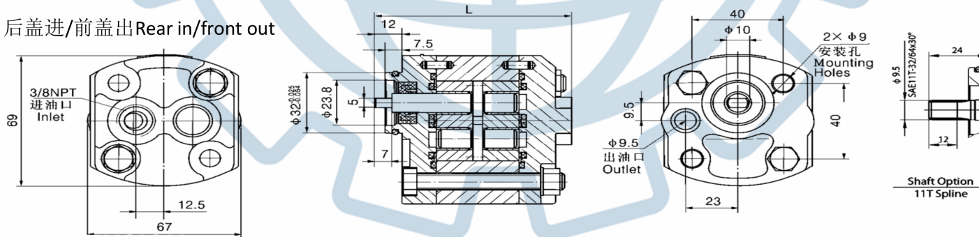
泵体进/后盖出 Side in/Rear out
